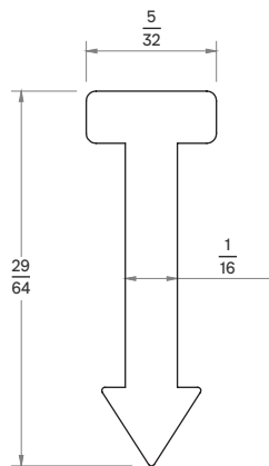
Type EM - 2"
