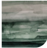
Sediment 'Forest'
