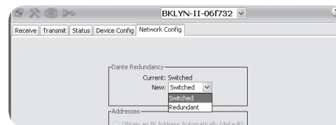
WING avec réseau DANTE redondant
