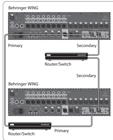
WING avec réseau DANTE redondant
