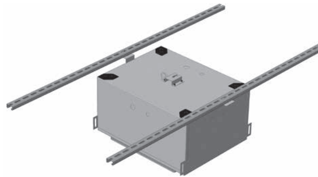
Rückendose zwischen Schienen montiert
