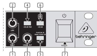
図 2.1: フロントパネル部
