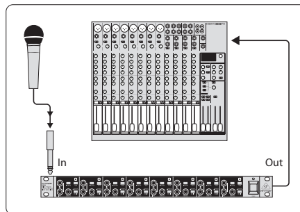
図 3.3: マイク接続
