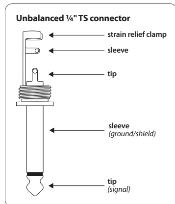
図 4.2: 6.3 mm TS コネクター
