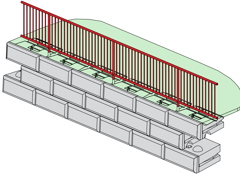
Zaun- oder Geländerpfosten mit Mörtel vergießen Feldkern in Block in zweiter Reihe
