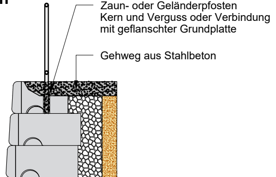
Gegen Verdrehung gesicherter Anschluss
