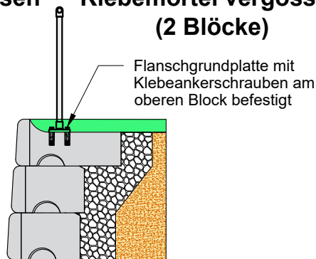
Steherflansch mit Bolzen am Betonblock angeschlossen
