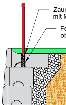
Eingebohrt und mit Klebemörtel vergossen (1 Block)
