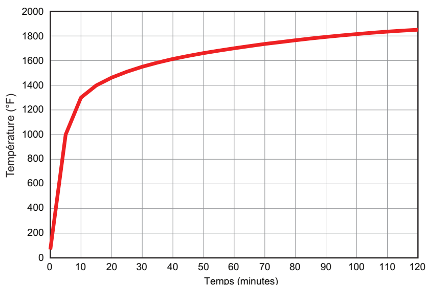
Temps standard - Courbe de la température pour le contrôle des essais au feu
