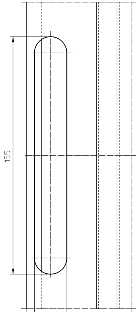
MILLING : FRAME
