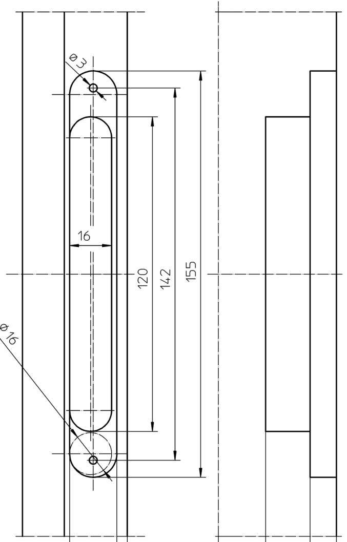
MILLING : DOOR LEAF
