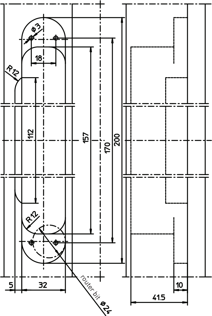
MILLING : FRAME
