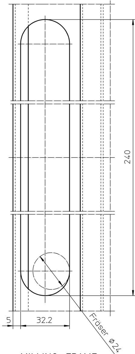
MILLING : FRAME
