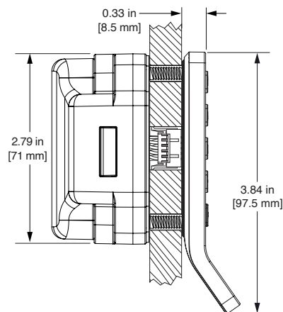
侧视图
