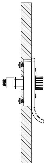
Vue latérale
