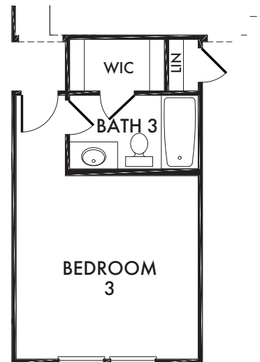
OPTIONAL BATH 3 OPT. #109
