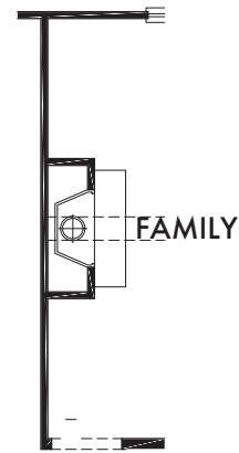
OPTIONAL FIREPLACE OPT. #301
