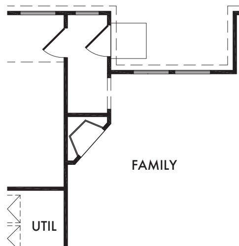
OPTIONAL FIREPLACE OPT. #300
